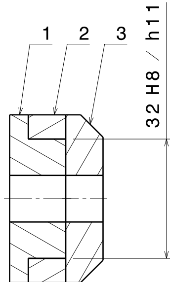
Coupe A-A
